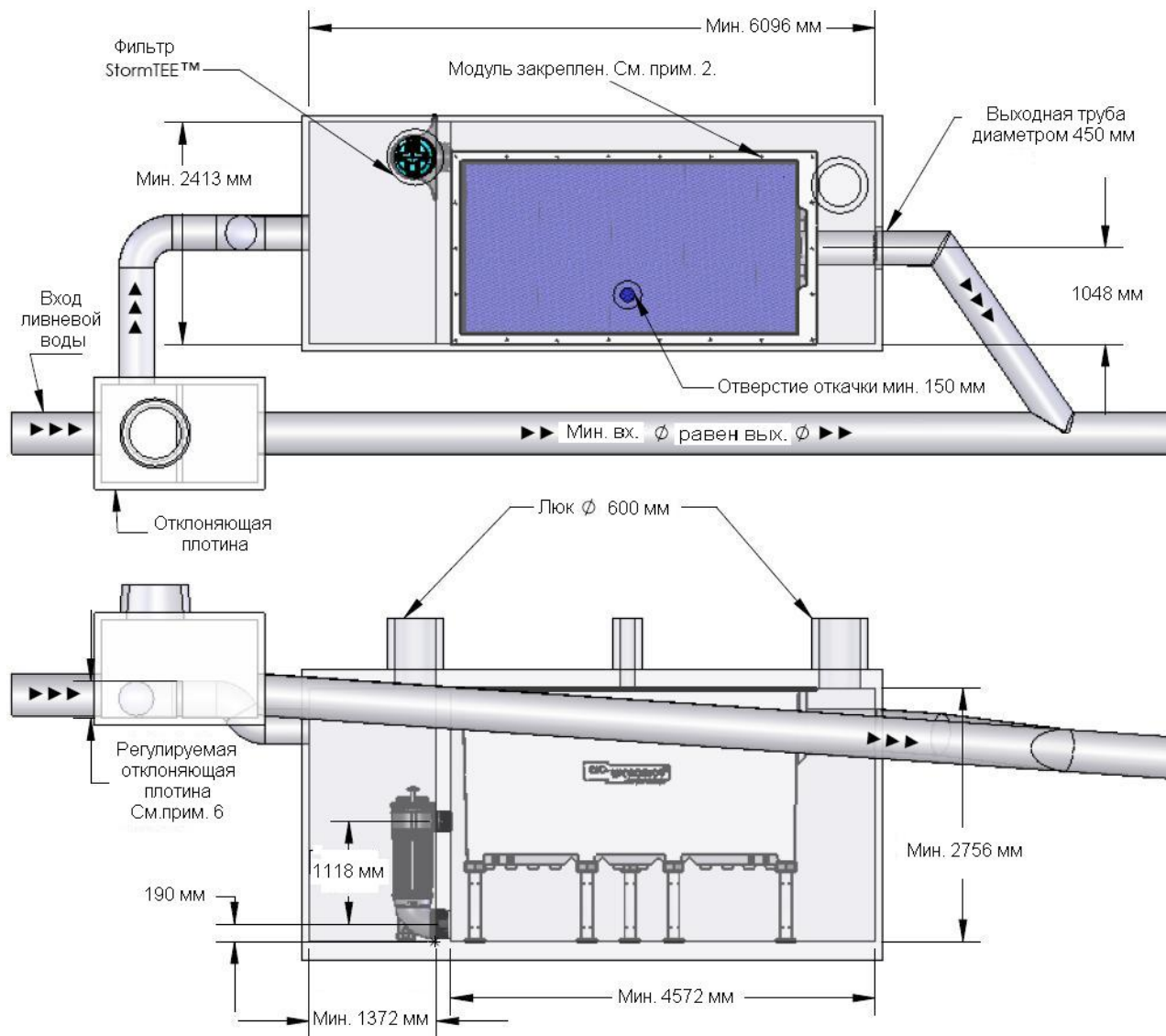
Рис.2. Общий вид системы очистки.
