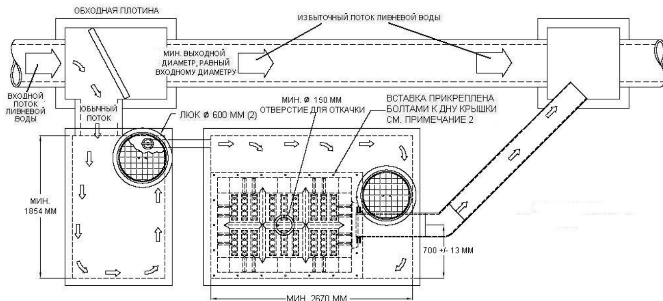
ВИД СВЕРХУ
